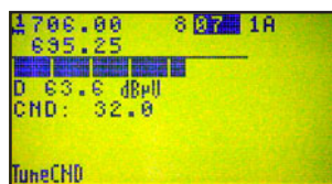
C/N-mätning A/D
